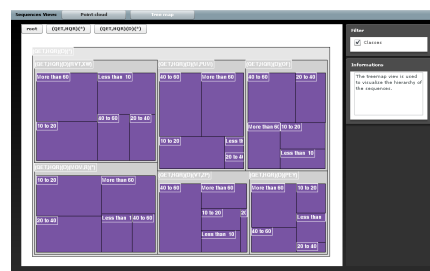
FIG. 3 – Treemap
