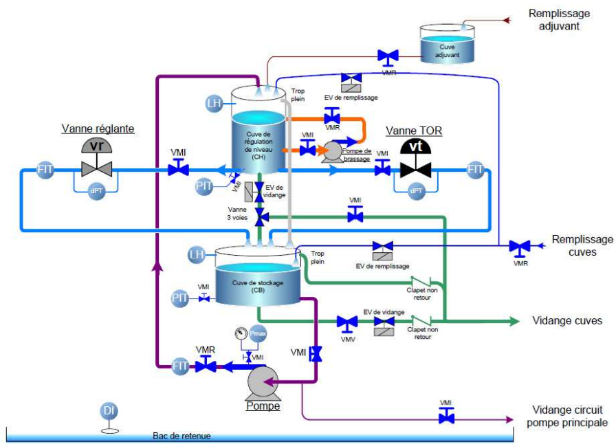
Figure 1 : Plan de circulation des fluides
