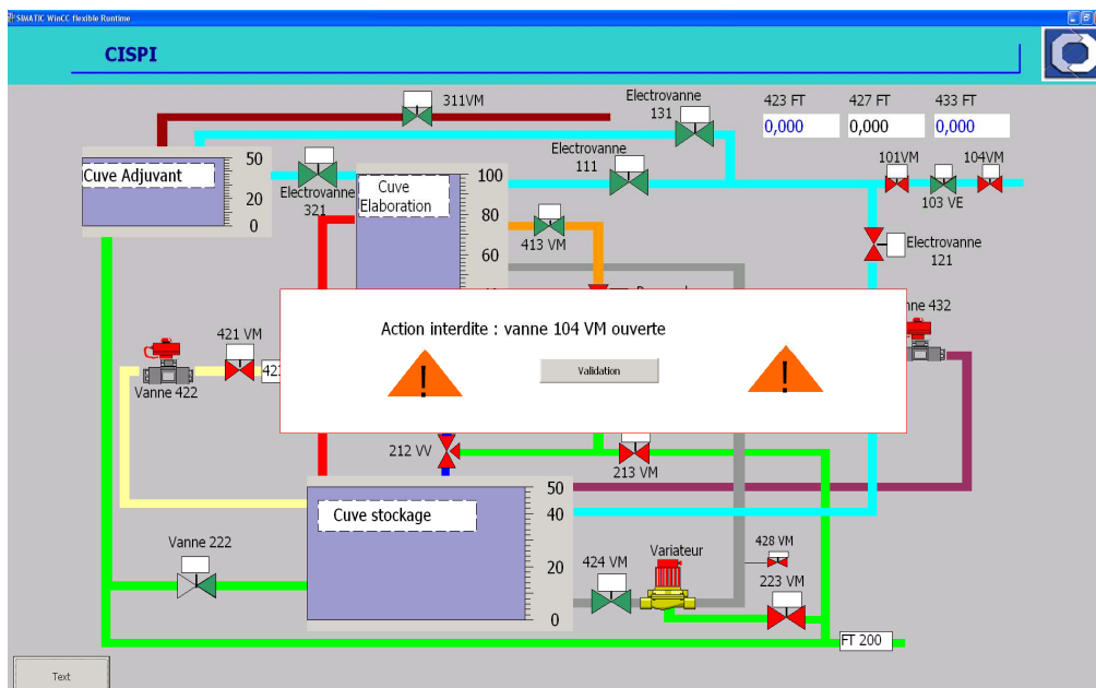
Figure 9 : Vue de l'écran de conduite indiquant qu'une action non conforme a été effectuée
