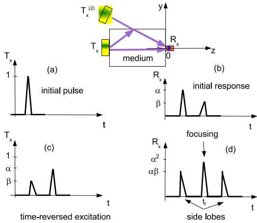
FIGURE 2 – Principe de focalisation par réciprocité : une excitation initiale (a) large bande T_x(t) se propage dans un milieu complexe dans lequel les échos additionnels (b) provenant des interfaces et des diffuseurs peuvent être associés à des sources virtuelles T_x^{(2)} . En appliquant le principe de réciprocité et de renversement temporel à la réponse R_x , la nouvelle excitation (c) renversée temporellement T_x(t) = R_x(-t) produit une nouvelle réponse R_x (TR-NEWS coda y_{TR}(t) ) possédant une focalisation spatio-temporelle au point z = 0; y = 0 , et au temps t = t_f . La propriété de symétrie de y_{TR}(t) par rapport au temps de focalisation t = t_f (présence de lobes latéraux) permet l'obtention d'une signature acoustique (localisée spatialement) associée à la nonlinéarité acoustique créée par la focalisation.
