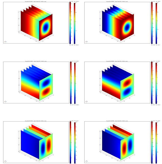
FIGURE 2 – Déformées modales (modes 1 à 6)
