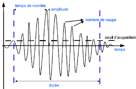
Figure 2 : Principaux paramètres temporels d'une salve d'émission acoustique.
