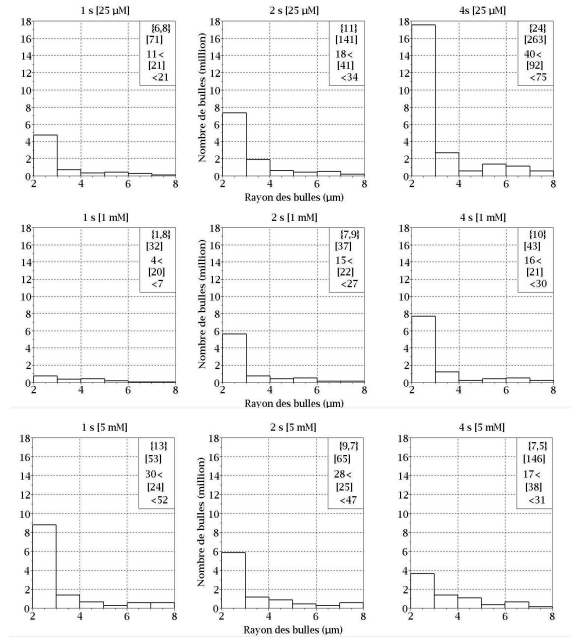
FIG. 8: Evolution de n(r) pour différentes concentrations de SDS (lignes) pour différentes durées (colonnes).
