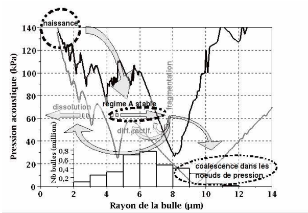
FIG. 3: Seuils de cavitation (courbe noire) et de croissance par diffusion rectifiée (courbe grise) ; distribution en taille des bulles et schéma d'évolution en régime A
