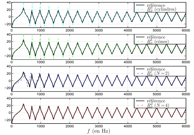
FIGURE 3 – Module (en dB) des impédances d'entrée calculées pour les profils \underline{R}_2^a (- - -), \underline{R}_2^b (- · - ·), \underline{R}_2^c (- · - ·) et \underline{R}_2^d (- · - ·), comparées à la référence (-).
