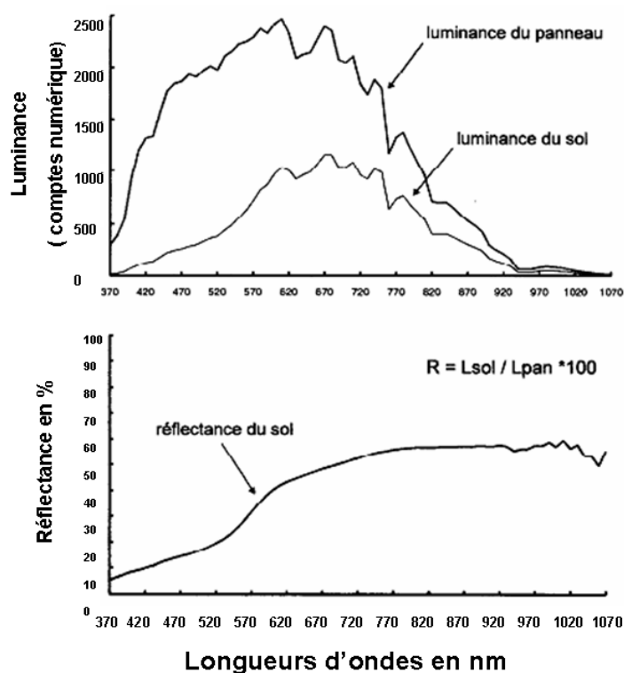
Figure 3 : Calcul de la réflectance à partir des luminances mesurées sur le sol et sur la cible de référence. Le spectre de réflectance est bruité dans le domaine spectral où la luminance est faible (970-1070 nm) ( Tiré de Escadafal et al. , 1993). Figure 3 : Computing reflectance from radiances measured over the soil and the reference panel. The reflectance spectrum is affected by noise in the spectral range where radiances are low ( 970-1070 nm) (data of Escadafal et al. , 1993).
