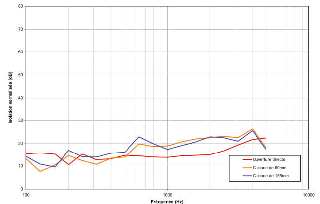
Figure 6 : Spectres d'isolation normalisée de la fenêtre ouverte avec un débit d'air d'environ 200 l/s sous 10 Pa, pour la fenêtre ouverte directement ou avec des chicanes de 80 et 155 mm
