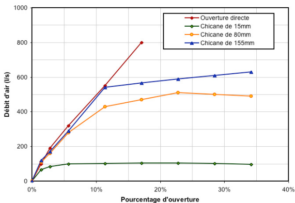
Figure 4 : Comparaison des débits d'air sous une pression de 10 Pa, pour différentes ouvertures de la fenêtre
