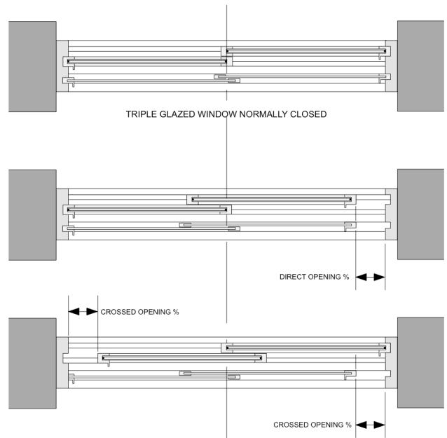
Figure 2 : Configurations d'ouverture (fermée, directe, en chicane) de la fenêtre coulissante à triple verre
