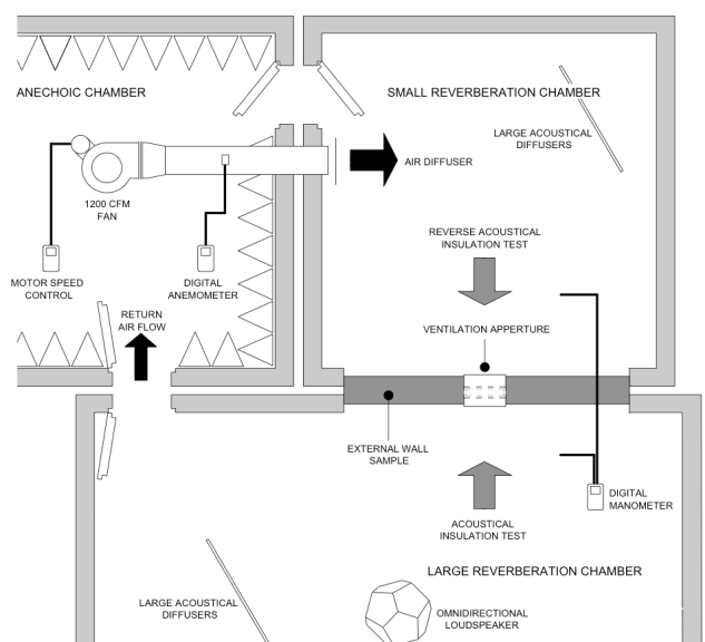
Figure 1 : Aménagement du laboratoire pour la réalisation des mesures d'isolation et de débits d'air
