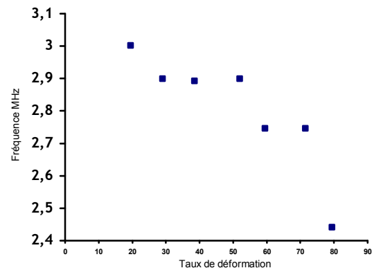
Figure 7: Fréquence en fonction du taux de déformation de l'Al 2024 pour une sonde de 2.25 MHz
