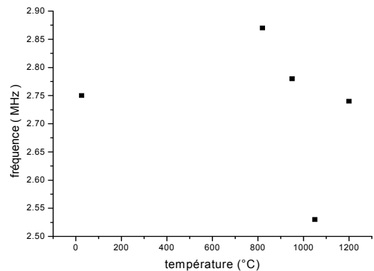
Figure 5: Fréquence en fonction du traitement thermique pour une sonde de 2.25 MHz
