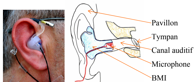
Figure 1 : Oreille équipée des deux microphones et position du microphone dans le BMI
