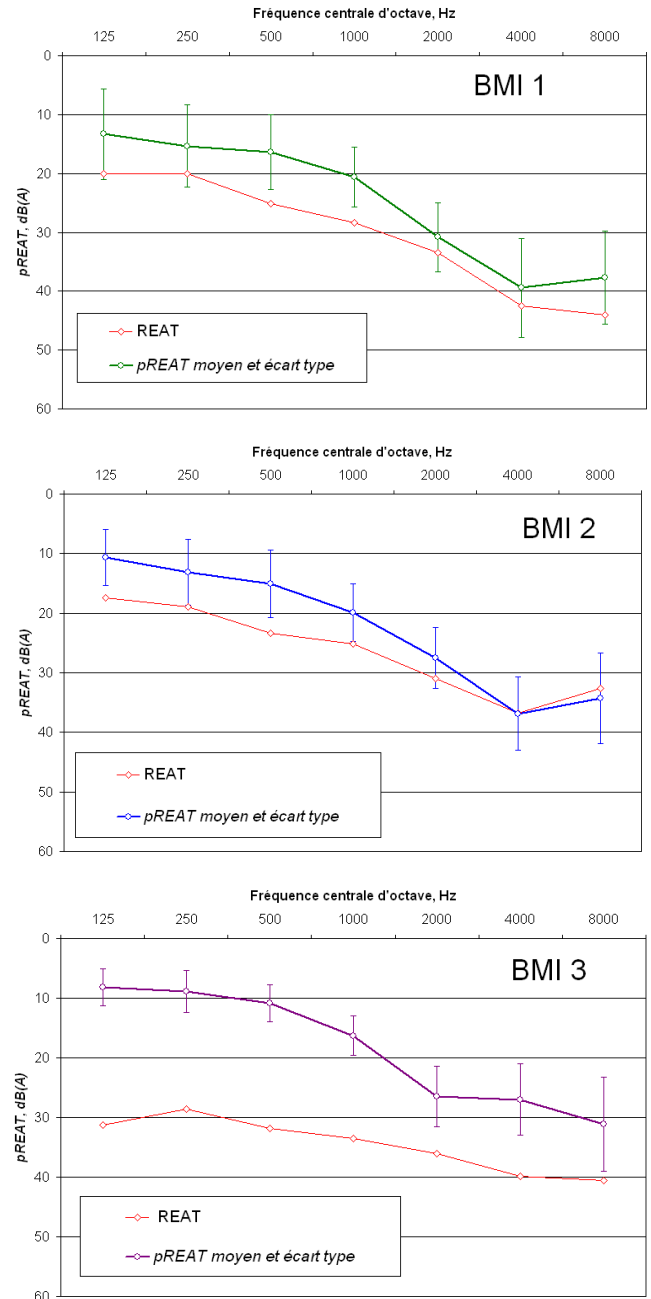
Figure 5 : Réduction corrigée du bruit (pREAT) comparée à l'affaiblissement acoustique établi en laboratoire (REAT) pour les trois BMI
