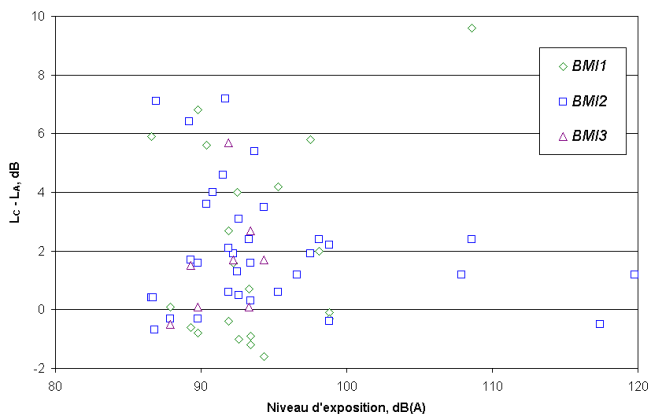
Figure 4 : Niveau d'exposition, fonction du L_C-L_A
