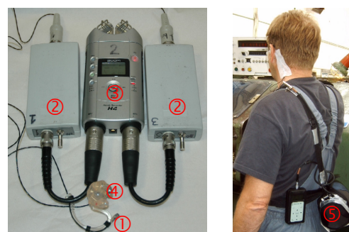
Figure 2 : Chaîne d'acquisition et équipement des sujets d'essai
