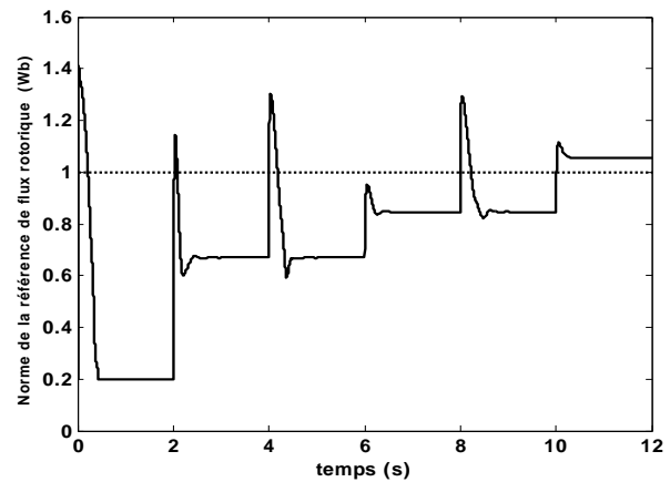
Fig 9: référence de la norme de flux rotorique en Wb. (Trait plein : régulateur à flux optimal, trait pointillé: régulateur à flux constant)
