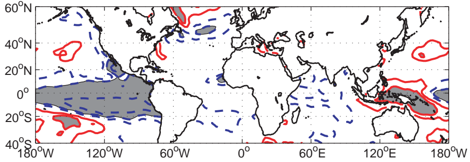
d): CC(SAH,SST): JAS 1991 2008
