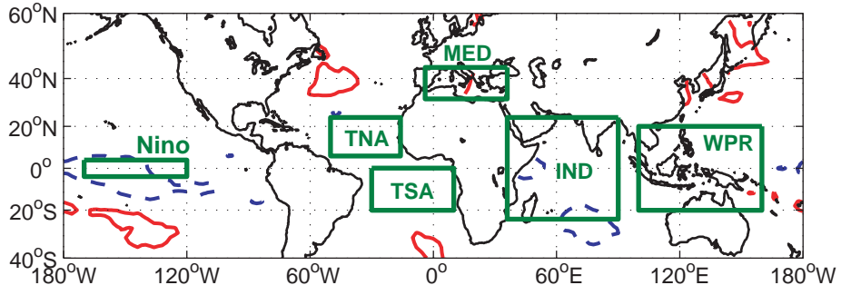
b): CC(SAH,SST): JAS 1950 1970
