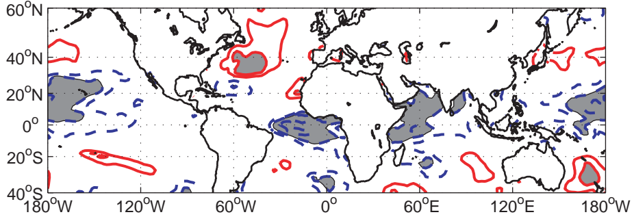
c): CC(SAH,SST): JAS 1971 1990
