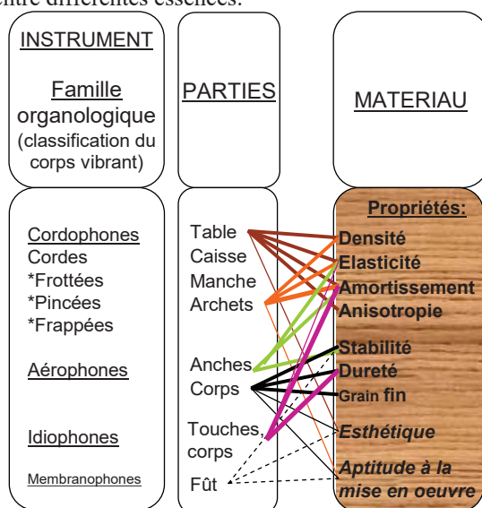
Figure 1: Vue schématique des propriétés physiques et technologiques des bois importantes selon les fonctions dans les instruments.
