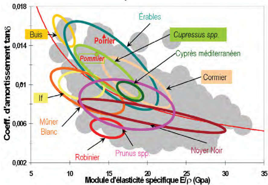
Figure 9: Gammes de variations de module d'élasticité spécifique et d'amortissement pour les essences listées dans le programme du CRPF pour lesquelles des données ont pu être trouvées. Nota : Quelques Prunus spp. et Acer spp. (= érables) supplémentaires ont été inclus. «Nuage » en gris : 330 espèces de bois (Résineux et Feuillus, tempérés et tropicaux) [Brémaud et al 2007].
