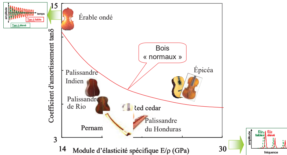
Figure 8: Comparaison des propriétés acoustiques élémentaires de bois représentatifs dans la fabrication d'instruments de musique classique Occidentale.
