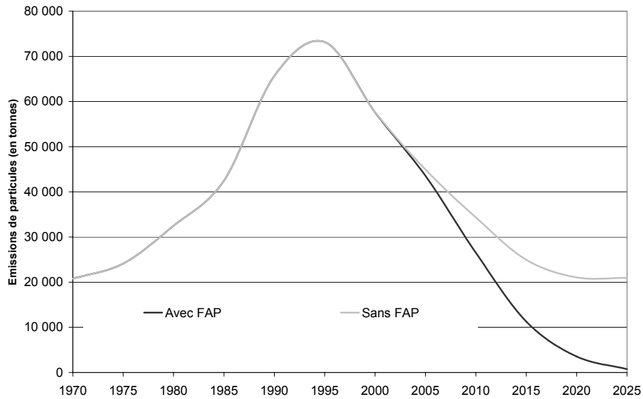
Figure 65 - Influence du filtre à particules sur les émissions en particules du parc routier français
