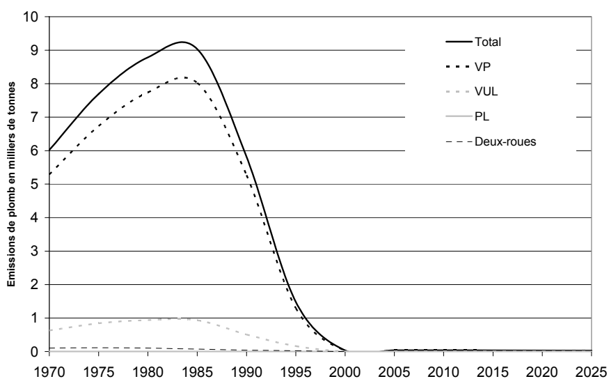
Figure 55 - Emissions de plomb du transport routier en France sur la période 1970-2025
