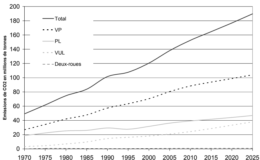
Figure 54 - Emissions de CO 2 du transport routier en France de 1970 à 2025
