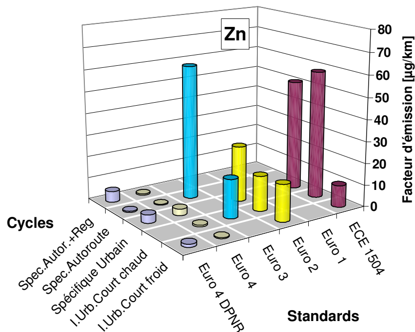
Figure 34: Emissions moyennes de zinc en µg/km selon la technologie pour les véhicules diesel (pre Euro à Euro4) testés sur des cycles réels (cycles Inrets).
