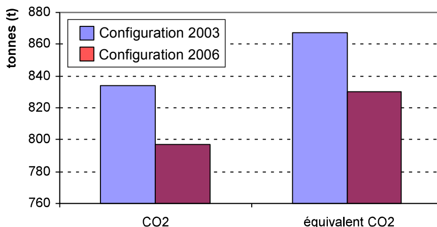
Figure 4-2 : L'évolution de CO 2 et d'équivalent CO 2
