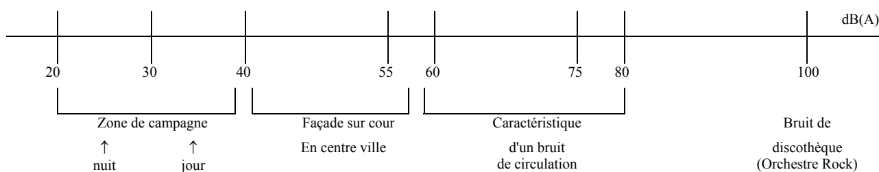
Figure 5-2 : Echelle des niveaux de bruit
