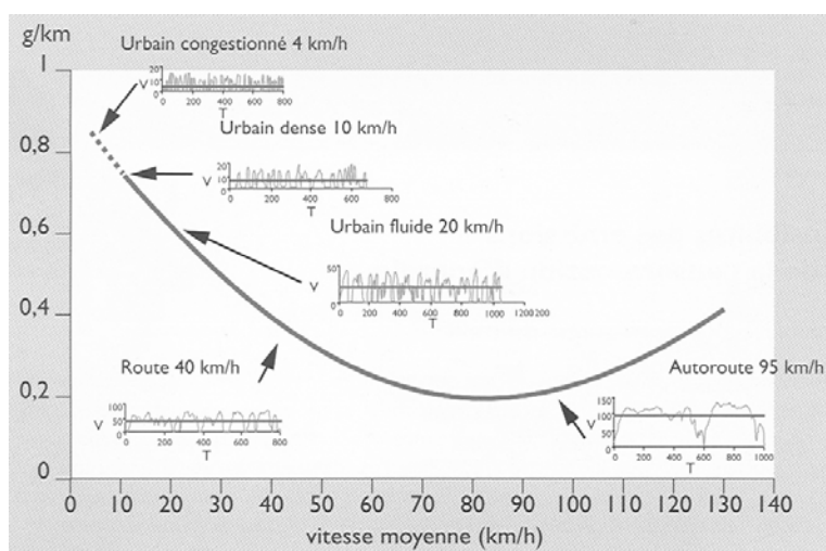
Figure 3-2 : Emission de NO x à chaud d'un véhicule essence catalysé en fonction de la vitesse moyenne et profils types de circulation V=f(T)
