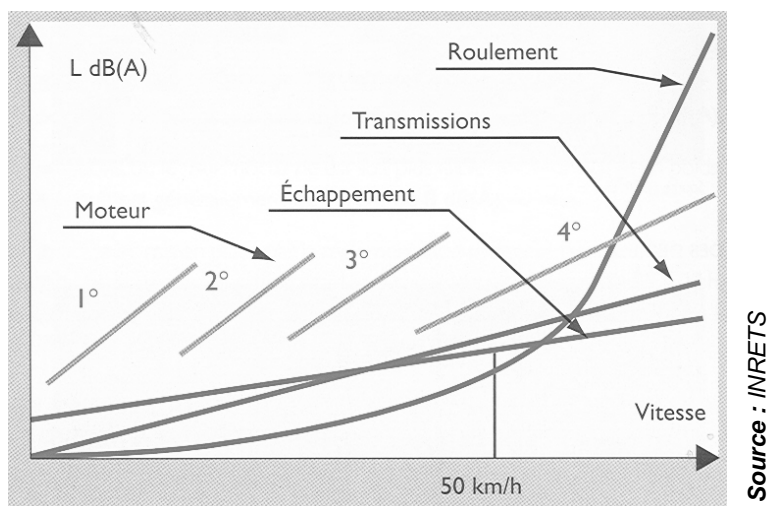
Figure 5-1 : Contribution des sources de bruit d'un véhicule selon sa vitesse
