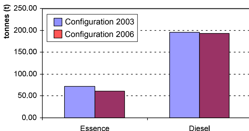
Figure 4-3 : Evolution journalière de la consommation de carburant sur le réseau d'influence du tronc commun A4-A86
