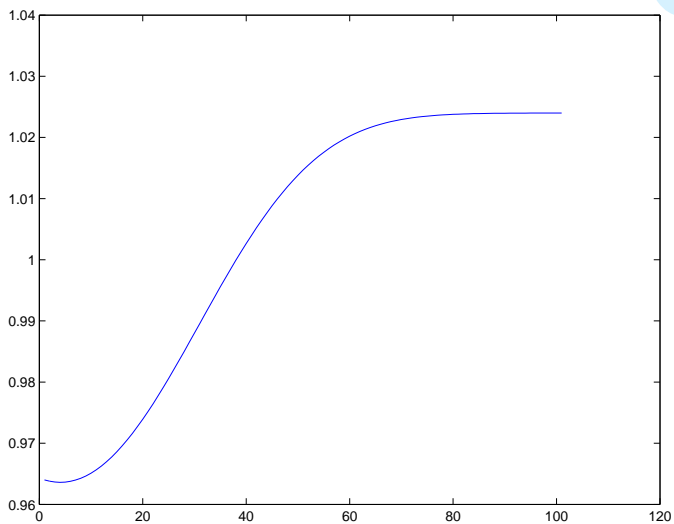
Figure 1. Diffusion
