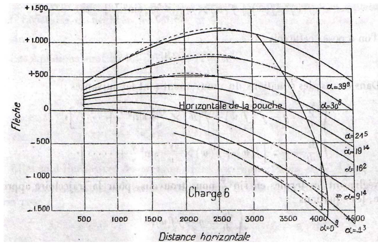
Fig.5 : Comparaison entre les courbes Krupp et les solutions approchées ([22], p.1001)
