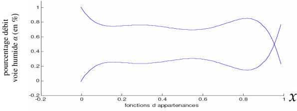
Fig. 7 : fonctions d'appartenance du modèle de température
