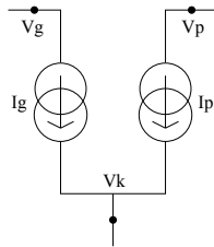
FIGURE 2 – Modèle de la triode
