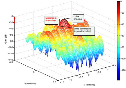
FIG. 5: Évaluation de l'influence des lobes secondaires en mesurant la différence en décibels entre le niveau du lobe principal et celui du lobe secondaire le plus important ( mssl ).
