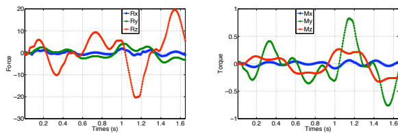
FIGURE 6 – Le torseur des efforts globaux en O
