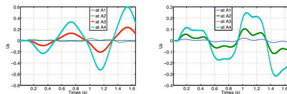
FIGURE 10 – Composantes u et w de \mathbf{u} aux points A_i .
