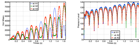
FIGURE 8 – Von Mises et niveau sonore aux points A_i
