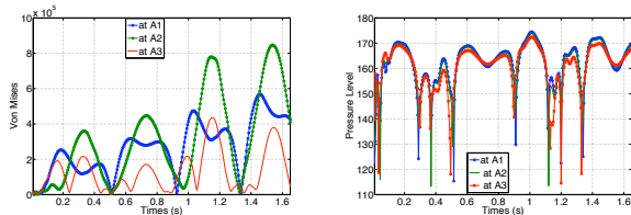
FIGURE 5 – Von Mises et niveau sonore aux points A_i
