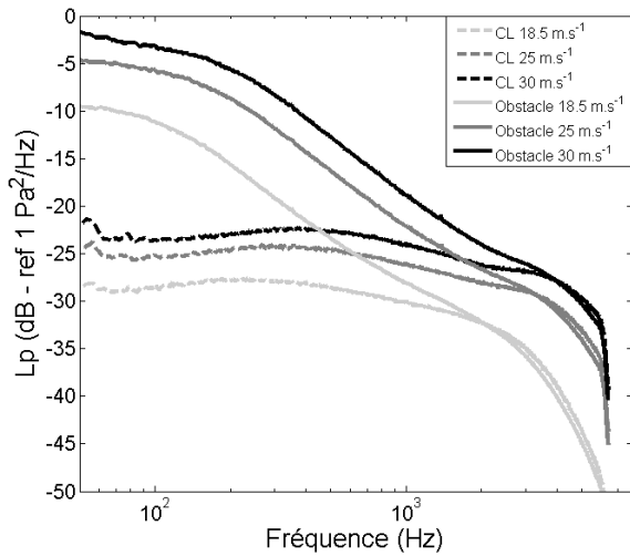
Figure 6 : Pression pariétale moyenne mesurée pour 3 vitesses d'écoulement (18.5, 25 et 30 m.s -1 ) avec et sans obstacle.
