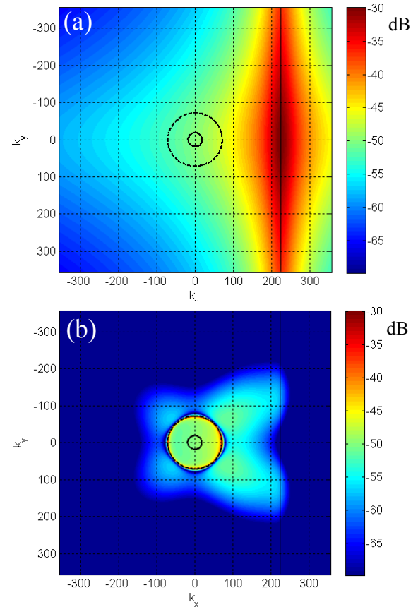
Figure 11 : (a) : énergie d'une CLT type Corcos ( U_\infty=40m/s , f=1kHz ) dans le domaine des nombres d'ondes.
