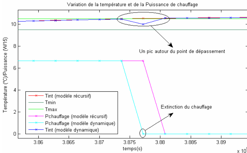
Figure 6 : Variation de la température et de la puissance de chauffage dans Simulink (6min)
