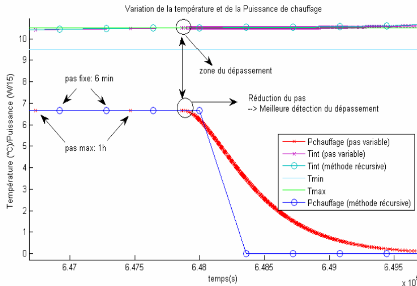
Figure 10 : Variation de la température et de la puissance de chauffage du modèle récursif (6min) et le modèle dynamique (pas variable 1s->1h)
