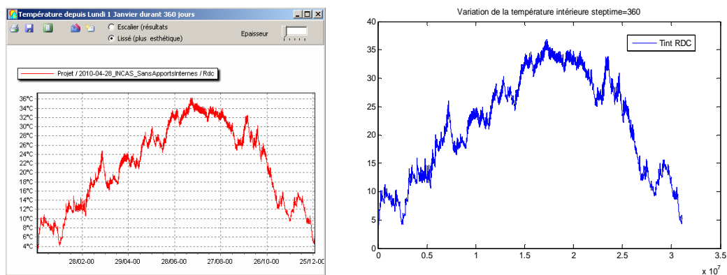
Figure 3 : Variation des températures simulées dans COMFIE (gauche) et dans MATLAB (droite)
