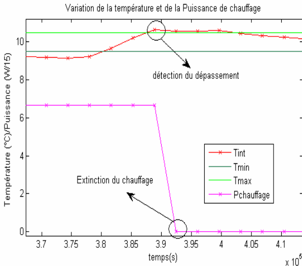
Figure 4 : Variation de la température et de la puissance du chauffage (pas 1h) dans MATLAB
