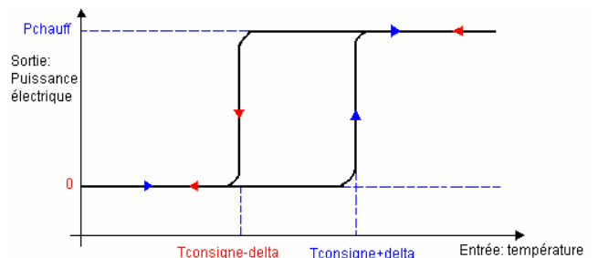
Figure 2 : Le principe de la commande du chauffage avec hystérésis
