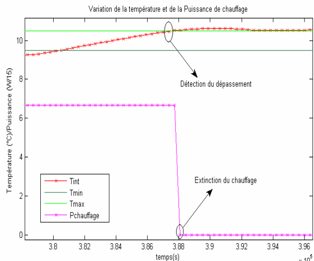
Figure 5 : Variation de la température et de la puissance du chauffage (pas 6min) dans MATLAB
