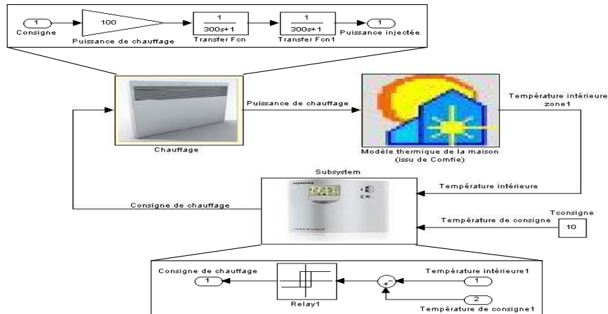
Figure 8 : Schéma de la simulation
