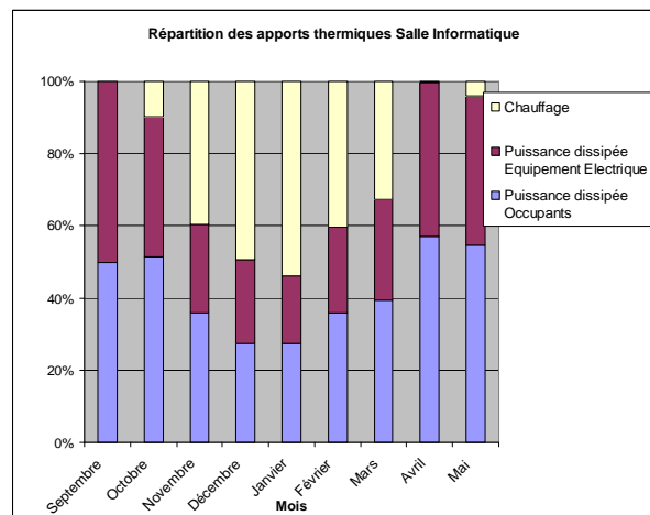
Figure 8 : Répartition énergétique des différentes sources thermiques
