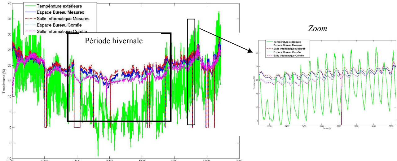
Figure 4 : comparaison de l'évolution des températures des zones Salle Informatique et Espace Bureau entre le 1 er Septembre 2009 et le 27 mai 2010
