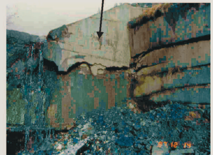
Fissuration d'une aile
