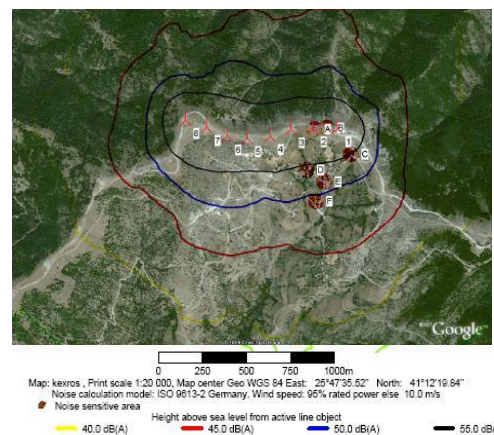
Figure 7. Niveaux de bruit de fonctionnement [selon la prévision du logiciel Wind PRO 1997]
