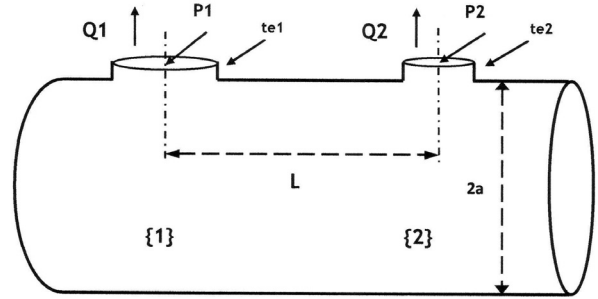
Figure 2 : surface interne d'une section de flûte à bec. Les hauteurs te_1 et te_2 sont dues aux épaisseurs acoustiques du corps; 2a = diamètre interne, S =section interne, L = distance des centres de {1} et {2}, 2b_1 et 2b_2 =diamètres respectifs, Q_1 et Q_2 =débits sortant, P_1 et P_2 =pressions de sortie.
