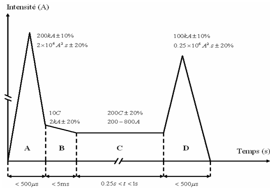
Figure 3: modèle de l'onde de courant associée à la foudre
