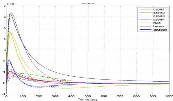
Figure 10 Réponse temporelle des courants dans chacun des câbles suite à une injection foudre
