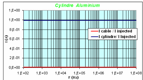
Figure 7: Redistribuition du courant dans le câble et le cylindre en aluminium
