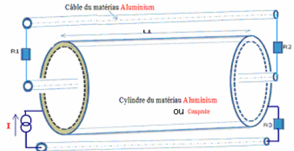
Figure 2 : dispositif décrit pour l'étude en mode rayonné
