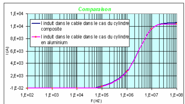
Figure 8: Courant induit sur le câble dans les cas du cylindre composite ou aluminium
