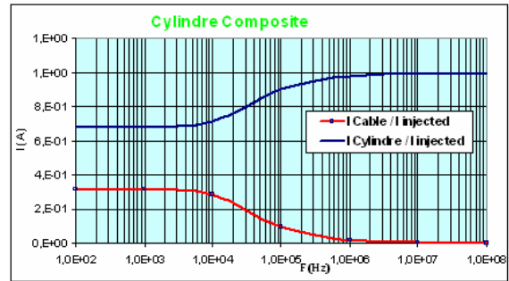
Figure 6: Redistribuition du courant dans le câble en aluminium et le cylindre en matériau composite
