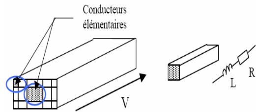
Figure 4: maillage unidirectionnel des câbles
