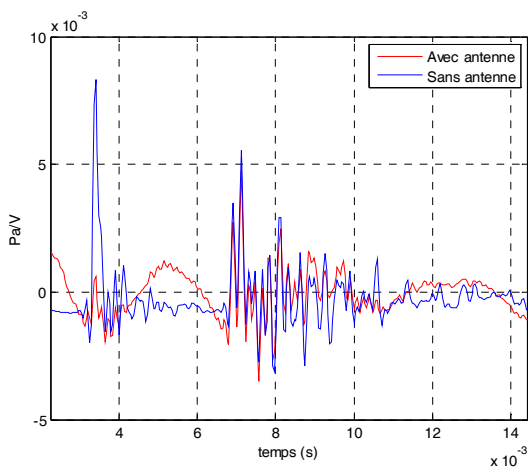
Figure 9 : Réponse impulsionnelle reçue par le capteur central de l'antenne (courbe bleu) et par le macro-capteur de l'antenne après traitement multipolaire (courbe rouge)
