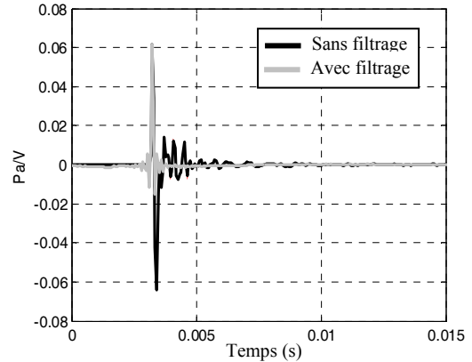
Figure 6 : Réponse impulsionnelle du système d'émission
