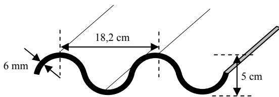
Figure 8 : Profil du relief ondulé étudié
