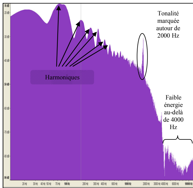
Figure 4 : Représentation 2D du spectre (intensité de chaque fréquence à un instant donné) pour la seconde 35 (figures 2 et 3) – illustration des caractéristiques d'un bruit d'avion
