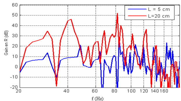
Figure 6 : Gain en indice d'affaiblissement acoustique R(dB) obtenu avec un contrôle actif complet simulé avec la méthode directe pour deux valeurs différentes de l'épaisseur L de la cavité d'air de la double plaque.
