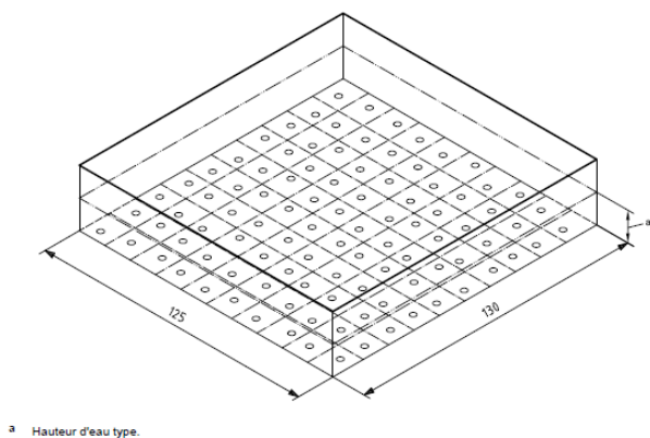
Figure A.1 — Représentation schématique du réservoir à embase perforée
