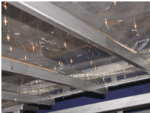
Figure 7 : Décrochement des gouttes en présence de buses individuelles (photo source VELUX)
