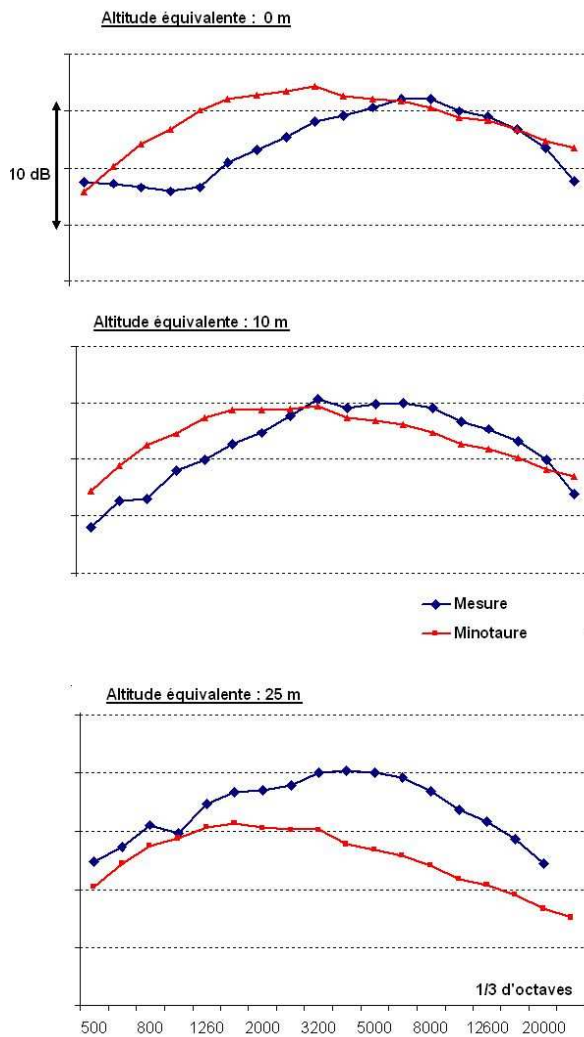
Figure 13 : VEGA à Colferro - Configuration carneau ouvert sans injection d'eau
