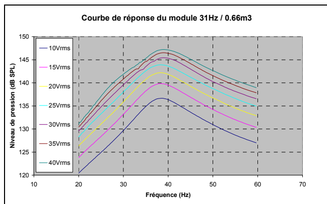
Figure 8 : courbe de réponse de l'actuateur 31.5Hz chargé par un volume clos de 0.66\text{m}^3
