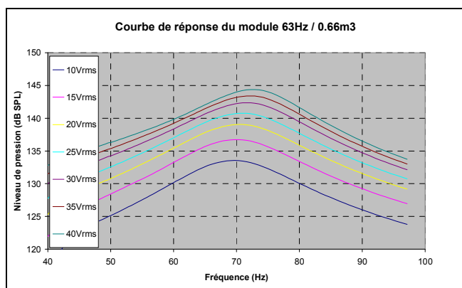
Figure 9 : courbe de réponse de l'actuateur 63Hz chargé par un volume clos de 0.66\text{m}^3
