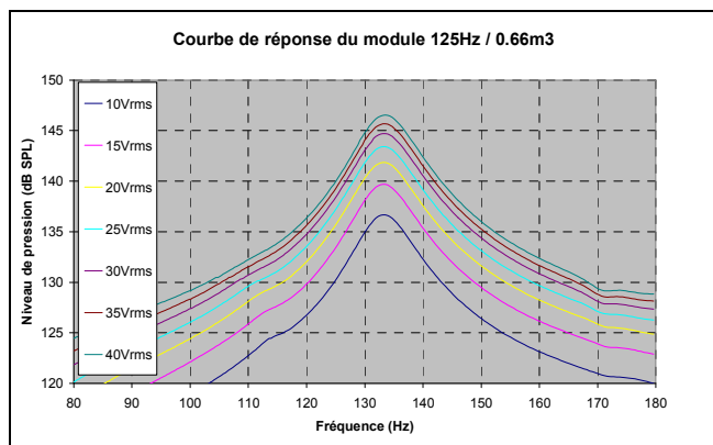
Figure 10 : courbe de réponse de l'actuateur 125Hz chargé par un volume clos de 0.66\text{m}^3
