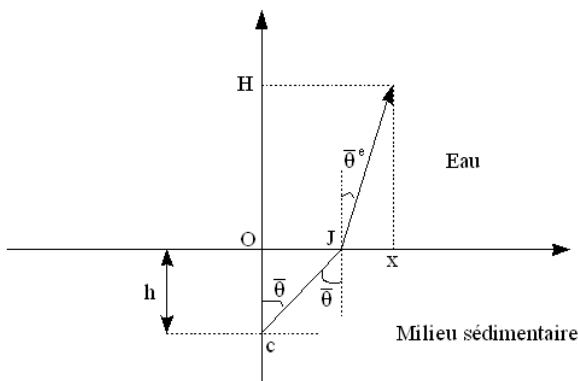
Figure 3 : Configuration pour la transmission dans l'eau de l'onde diffusée par le cylindre dans le sédiment. [4].
