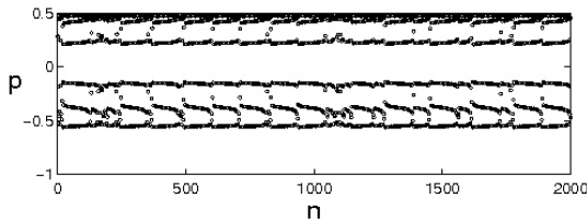
FIG. 3: Valeurs de la pression pour 2000 itérations. On a l'impression d'une succession de régimes à 6 états, la figure 4 montrant que le régime est chaotique. ( \gamma = 0,4664 \zeta = 0,8 \lambda = 0,95 )
