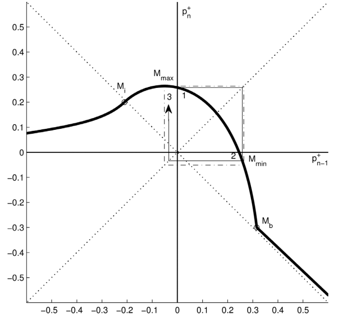
FIG. 2: Fonction non linéaire reliant l'onde aller à l'instant t , notée p_n^+ à l'onde aller à l'instant t - 2l/c , p_{n-1}^+ . Les paramètres sont \gamma = 0,4 \zeta = 0,8 \lambda = 0,95 . En pointillé le carré limité par les valeurs f_{min} et f_{max} pour l'abscisse et l'ordonnée. Nous montrons aussi le début d'une itération pour une condition initiale donnée (points 1, 2, 3)
