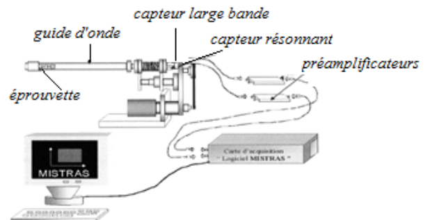
Figure 4 : Dispositif d'émission acoustique de l'installation
