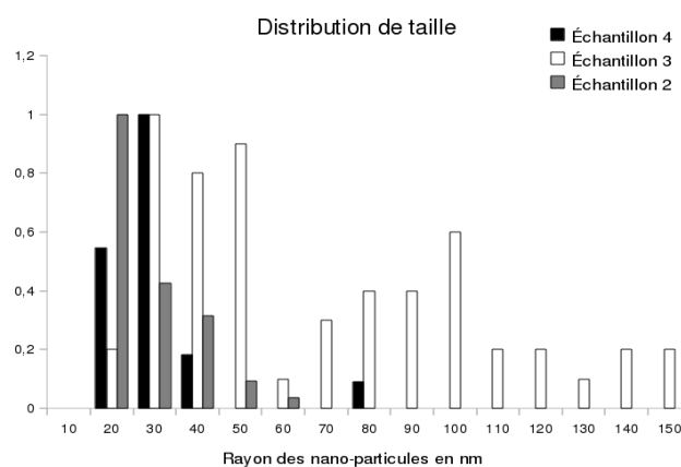
FIG. 2 : Distribution de taille des nano-particules.
