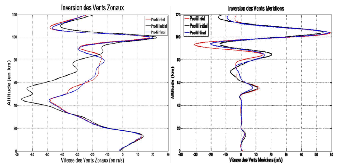
Figure 4. Profils de vents zonaux et méridiens obtenus lors d'une expérience jumelle
