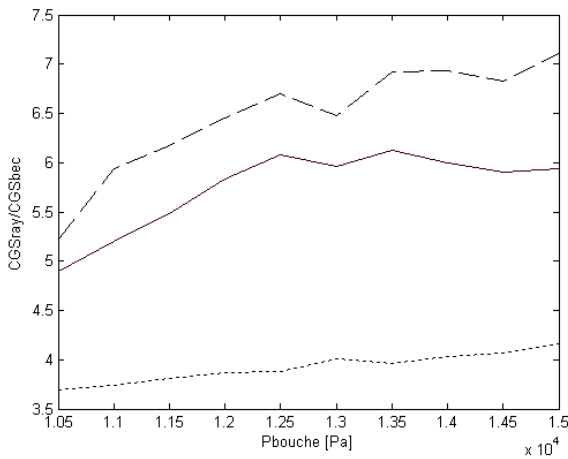
Figure 4 : Rapport des CGS de la pression rayonnée et de la pression mesurée dans le bec ( P_{\text{bec}} ), en fonction de la surpression dans la bouche ( P_{\text{bouche}} ).
