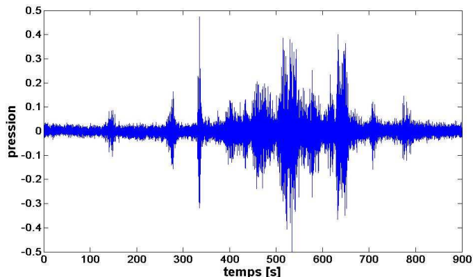
Figure 5 : signal temporel filtré à 0,5 Hz, série B
