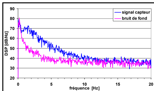
Figure 6 : spectre lissé, signal brut + bruit de fond
