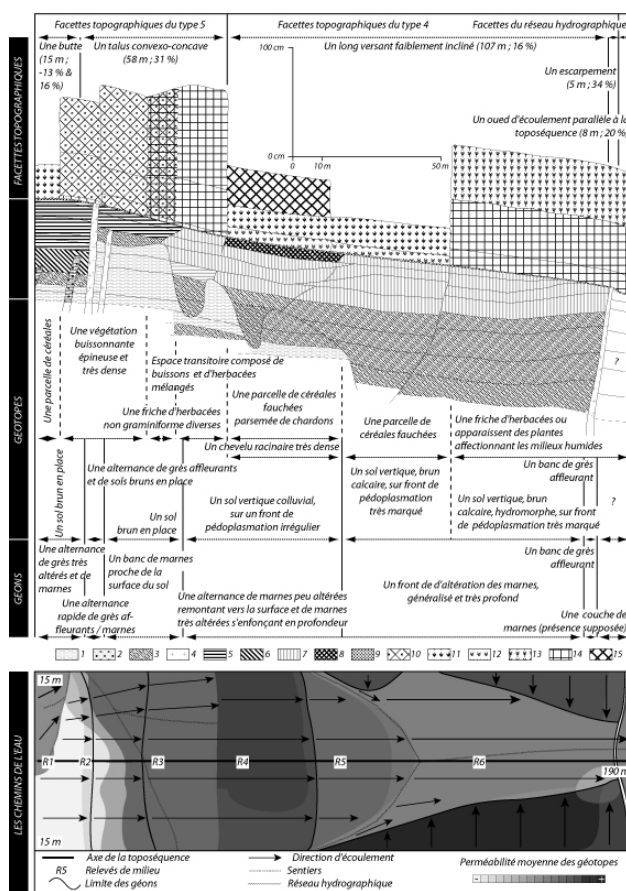
Figure 4 : caractéristiques et répartition des géons et géotopes le long d'une toposéquence. Légende : 1 – alté-tanolite ; 2 – isaltérite gréseux, 3 – isaltérite marneux, 3 – alté-récolite, 5 – brunichron, 6 – isa-brunichron, 7 – entaféro-vertichron, 8 – grumorhize, 9 – dermilite, 10 – nanophyton, 11 – nécro-gramen, 12 – gramen, 13 – kortode spinescent, 14 – kortodes, 15 – nanophyto-gramen.
