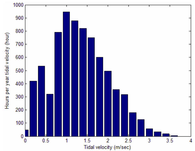
Fig. 13. Raz de Sein site tidal histogram.
