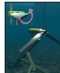
Fig. 6. The 3 (E-tide) blades options [© Strøm AS].
