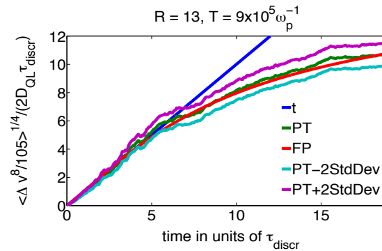
(d) \mathfrak{M}_8
