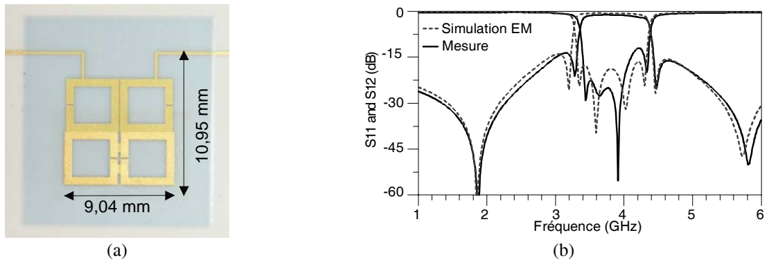
Figure 4 : (a) Photographie du filtre passe-bande DBR multicouche d'ordre 4. (b) Simulation et résultats de mesure du filtre.
