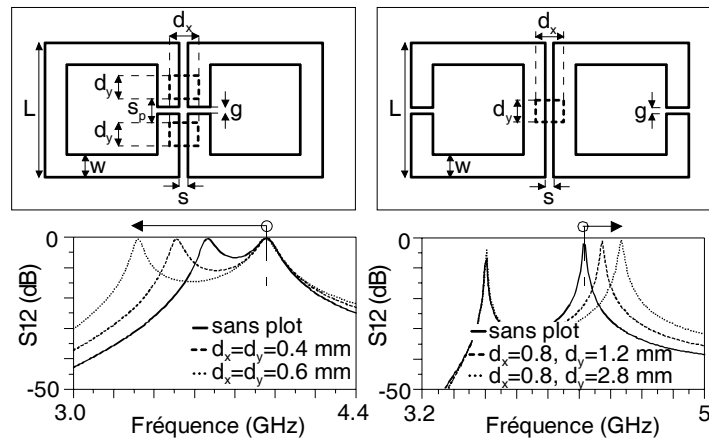
Figure 2 : Configurations de couplage avec et sans plots métalliques flottants.
