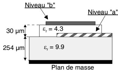
Figure 1 : Structure multicouche.
