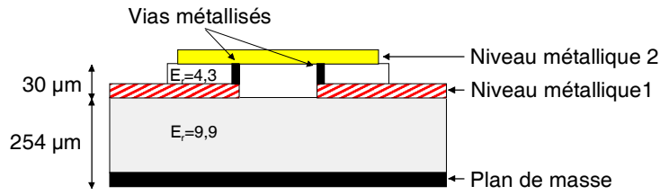
Figure 1 : Structure multicouche.
