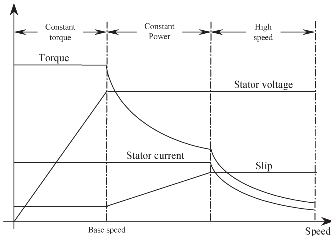
Fig. 6. IM characteristics.
